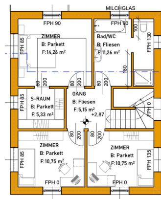
OG Haus 1
